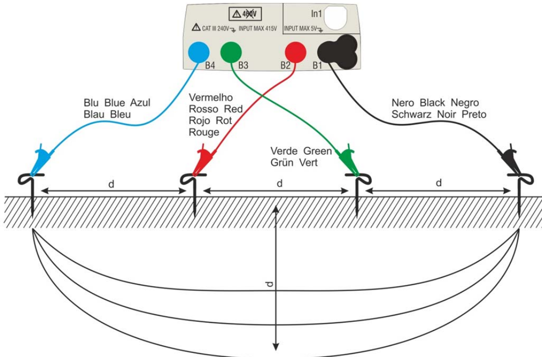
Abb. 31: Messung des spezifischen Erdwiderstandes
