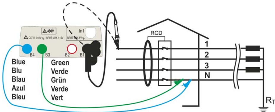
Abb. 15: Geräteanschluss zum 400V + N (no PE) dreiphasigen Test des RCD-Schutzschalters mittels Einzelkabeln und Tastkopf ( nicht für RCD Typ B )
